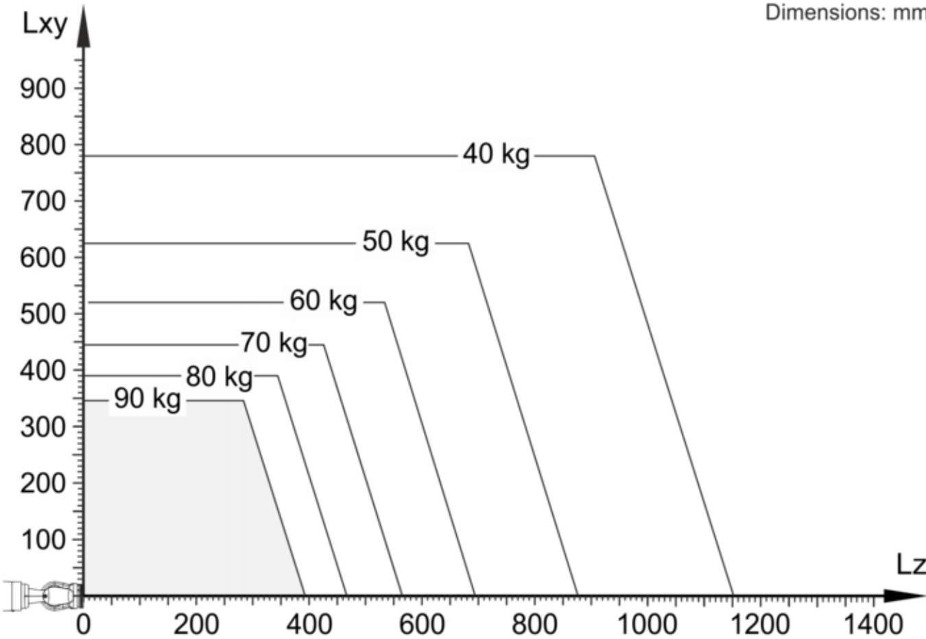
KR QUANTEC extra 负载能力图表，负载能力 90 kg
